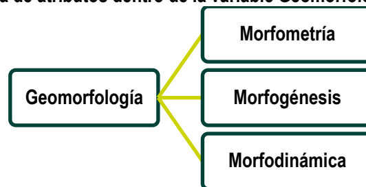
Figura 0.17 Diagrama de atributos dentro de la variable Geomorfología
