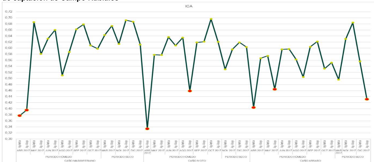
Figura 0.21 Resultados ICA multitemporal para los Caños Masisiferiano, Ivoto y Arrabo en los puntos de captación de Campo Rubiales
