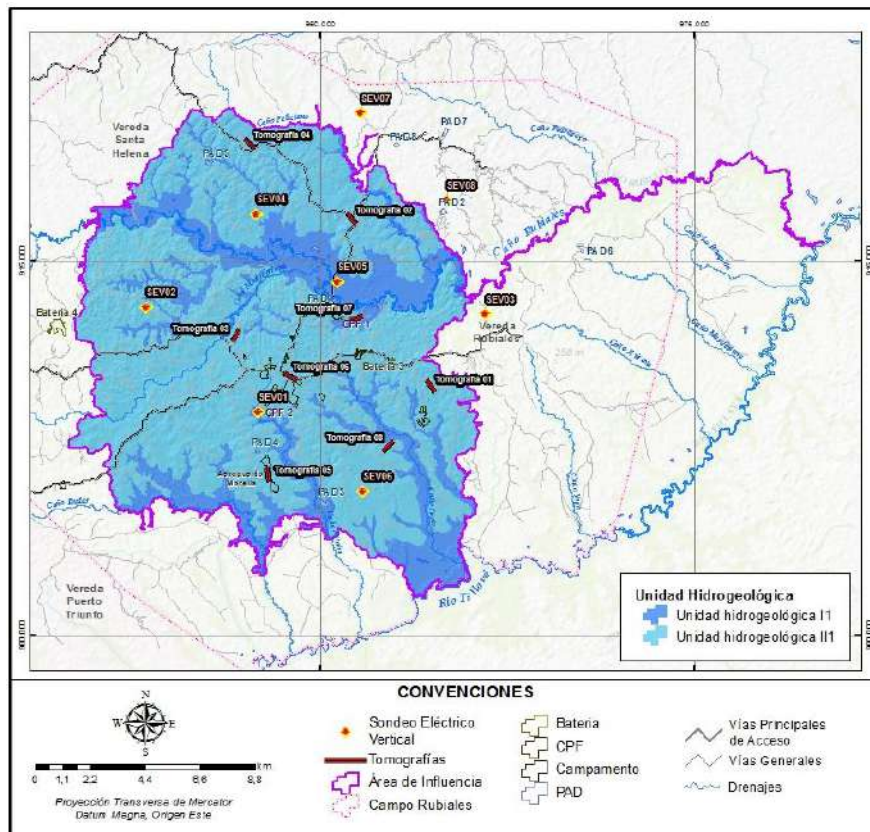
Figura 0.26 Ubicación espacial de los SEV y las tomografías eléctricas ejecutadas en el área de influencia
