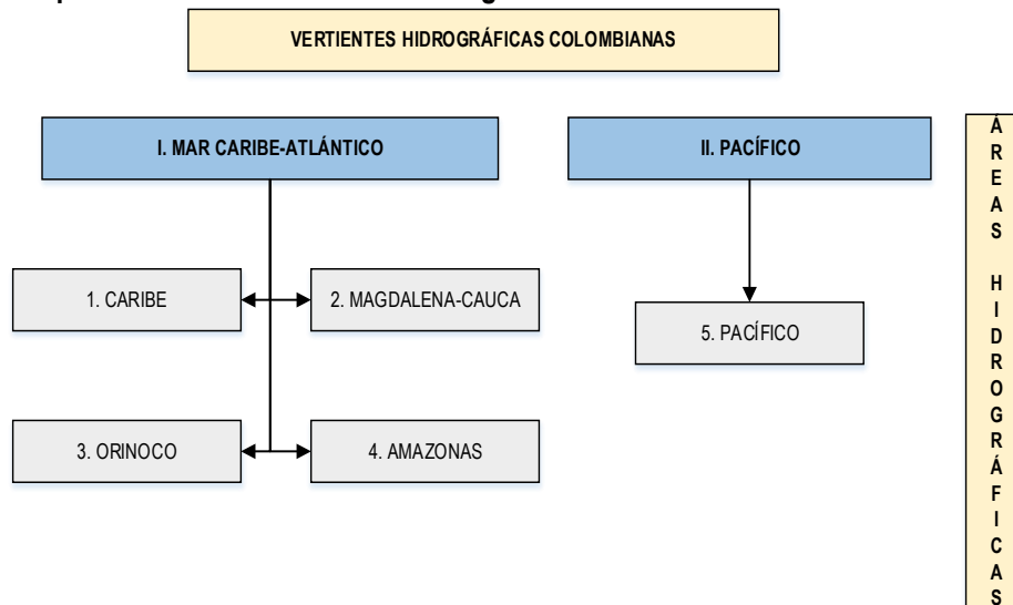
Figura 0.19 Esquema General Zonificación Hidrográfica de Colombia
