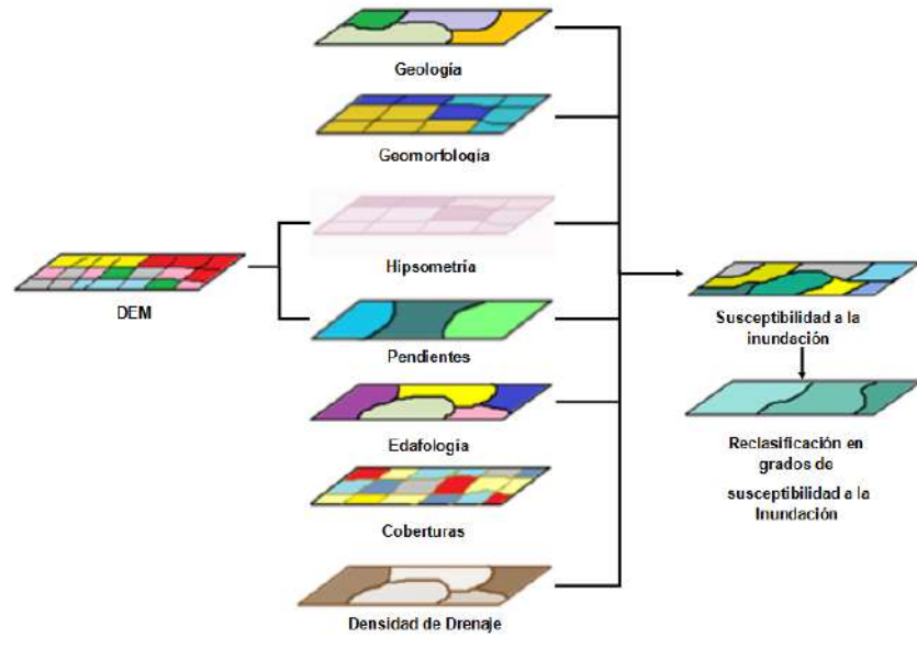
Figura 0.20 Procesos en el modelamiento espacial de la Susceptibilidad a la Inundación
