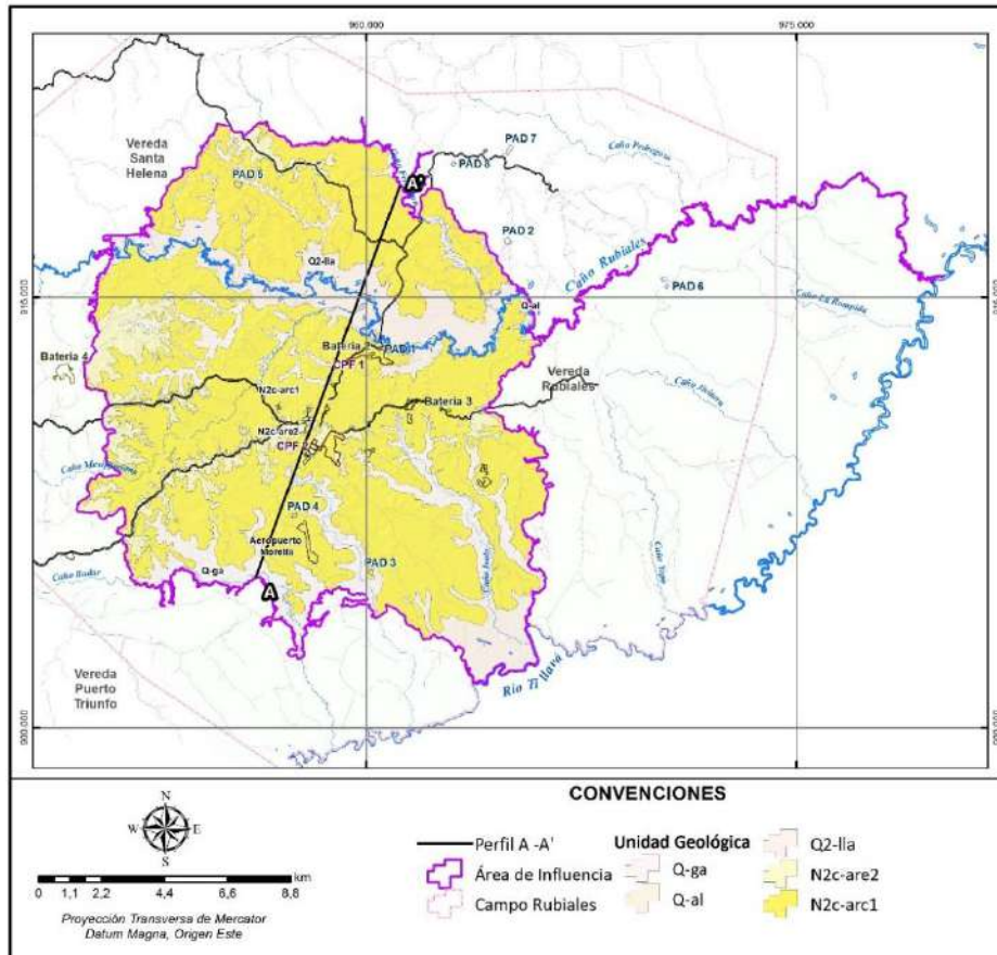
Figura 0.16 Mapa geológico del área de influencia
