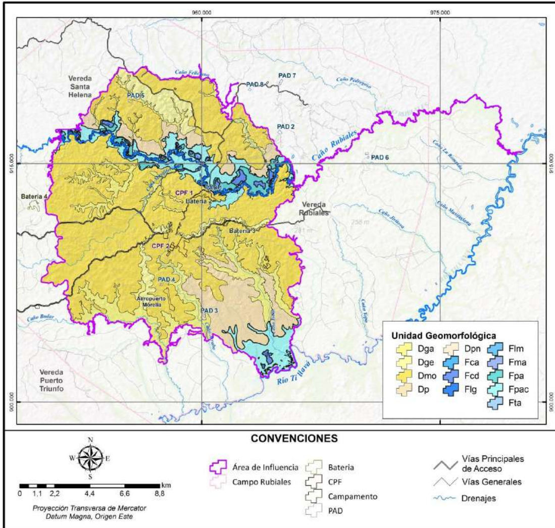
Figura 0.18 Geomorfología del área de influencia
