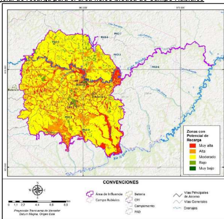
Figura 0.23 Potencial de recarga para el área físico biótica de Campo Rubiales
