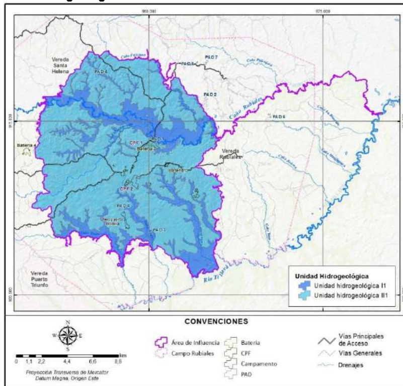
Figura 0.22 Unidades hidrogeológicas identificadas en el área de influencia físico biótica
