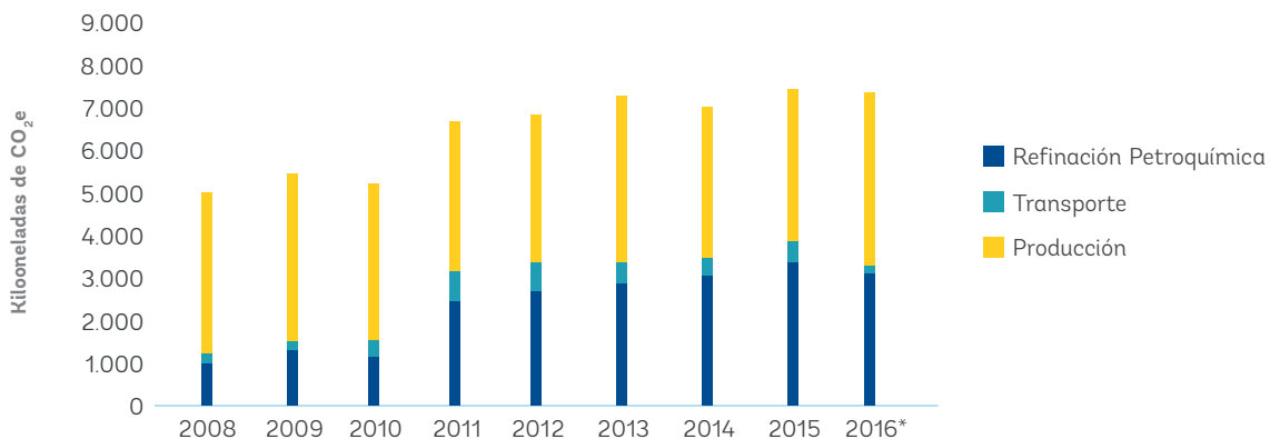
(G4-EN15) Gráfico 70. Emisiones directas por proceso operativo - Kilotoneladas de CO 2 e
