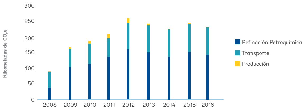
(G4-EN16) Gráfico 71. Emisiones directas por proceso operativo - Kilotoneladas de CO 2
