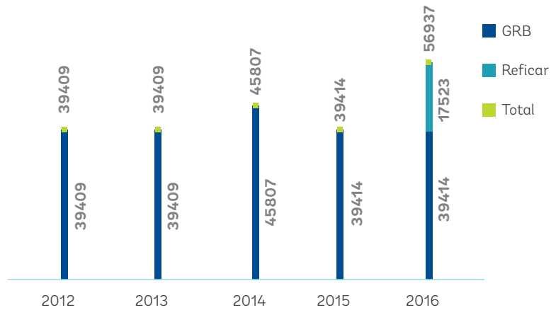
Gráfico 56. Demanda de energía para refinación (2012 - 2016)*
